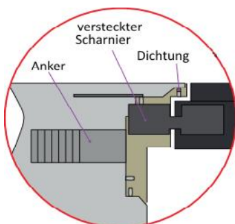
Schnitt des Türrahmens nach außen öffnend Variante B
